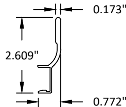
38 OPTIONAL 5/8" RISER 6063-T5
