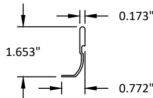
37 OPTIONAL 5/8" RISER ADD ON 6063-T5
