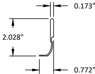
35 OPTIONAL 1" RISER ADD ON 6063-T5
